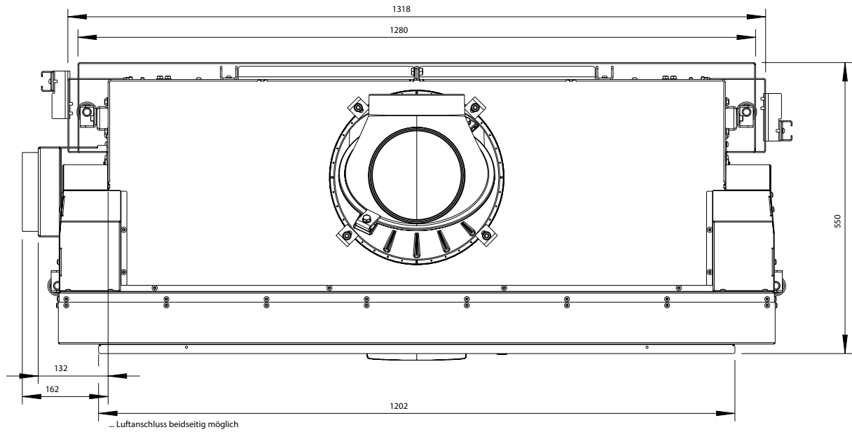
Maßstab 1:10
