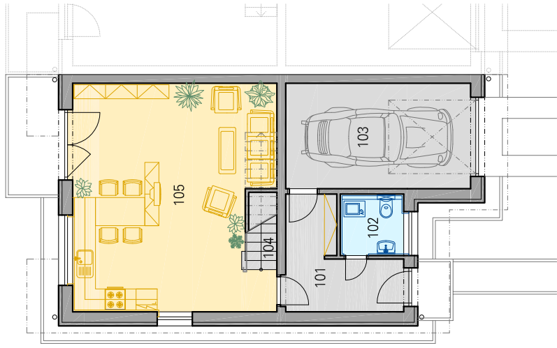
PŮDORYS 1.NP
