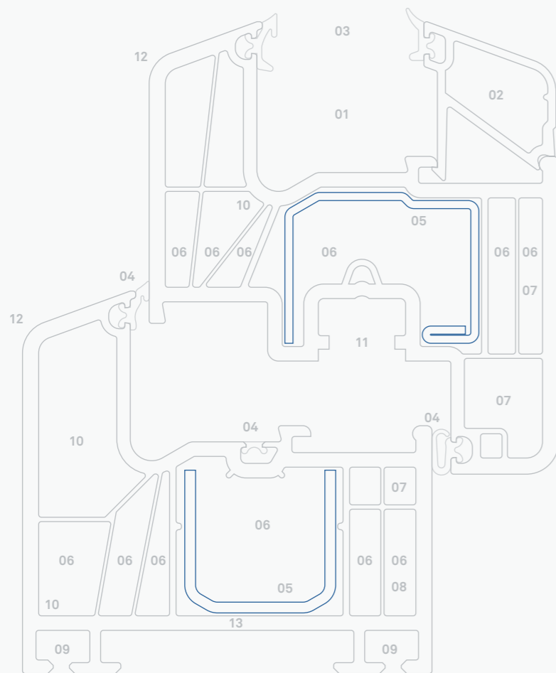
Prestige klasický profil I 76.6 C2 Dorazové těsnění (AD)
