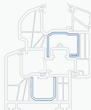
Prestige aktuální profil I 76.6 C4 Středové těsnění (MD)
